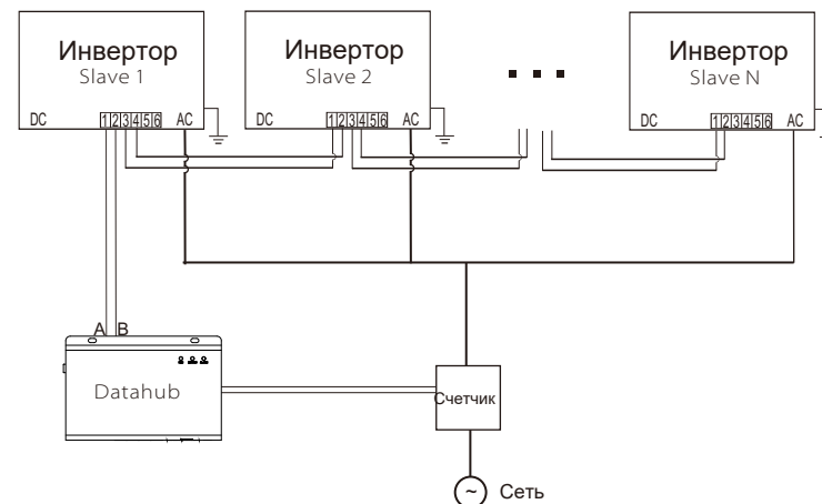
Diagram B: подключение через Dathub
